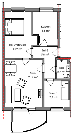
Eksisterende forhold 1:200
