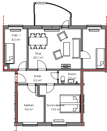
Eksisterende forhold 1:200
