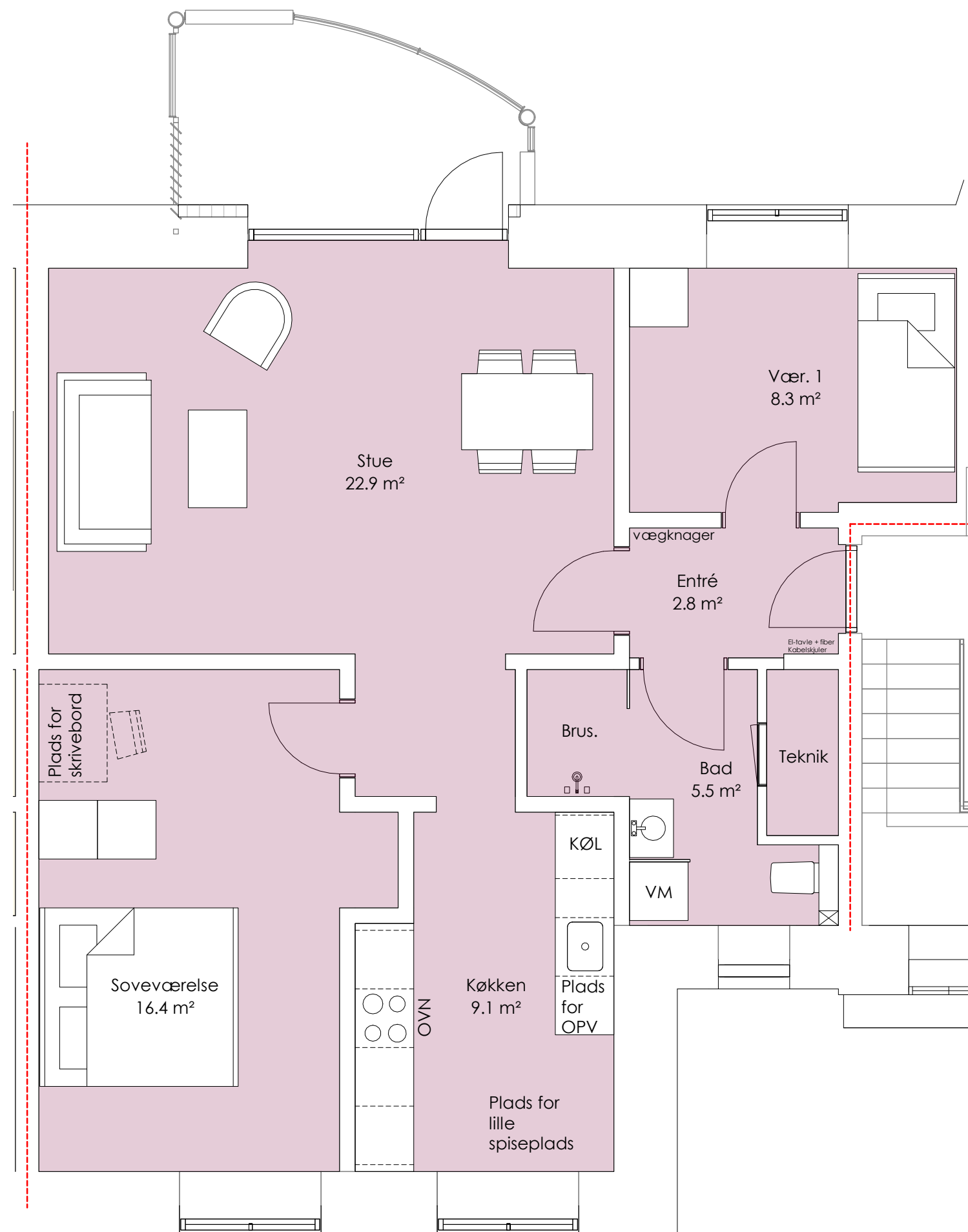
Fremtidige forhold
