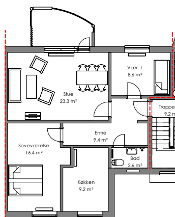
Eksisterende forhold 1:200
