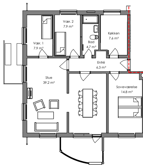
Eksisterende forhold 1:200
