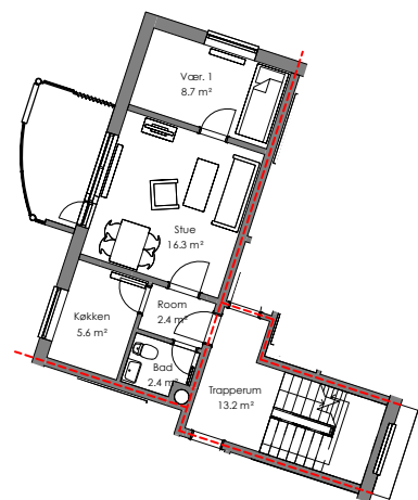
Eksisterende forhold 1:200
