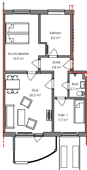
Eksisterende forhold 1:200
