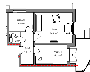
Eksisterende forhold 1:200
