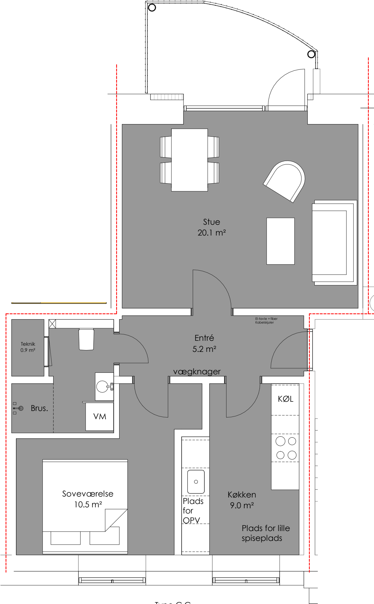
Type C.C 3 vær. H.C.Ø.V nr. 114 St-1-2. Tv
