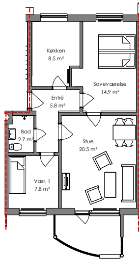
Eksisterende forhold 1:200
