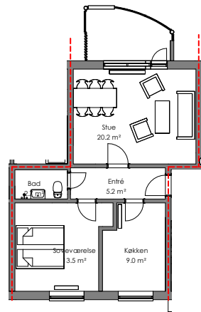
Eksisterende forhold 1:200
