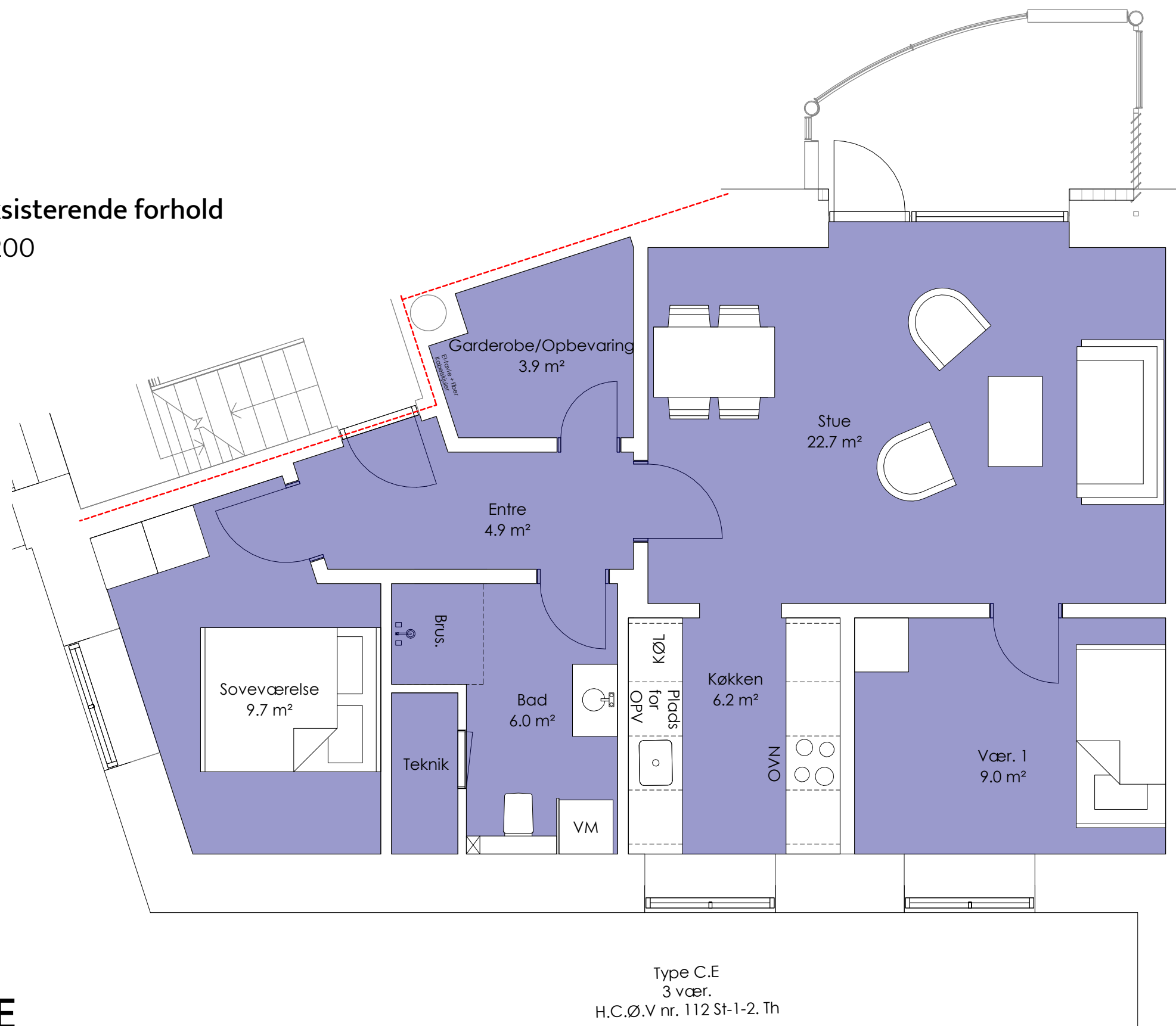
Fremtidige forhold
