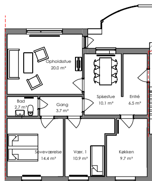
Eksisterende forhold 1:200
